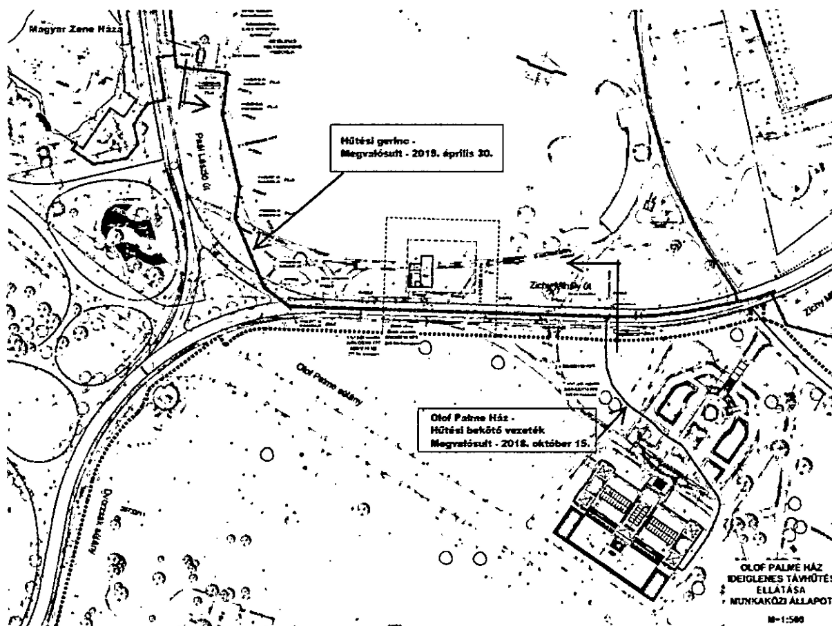
2. ábra Olof Palme Ház – Hűtési gerinc vezeték nyomvonal
