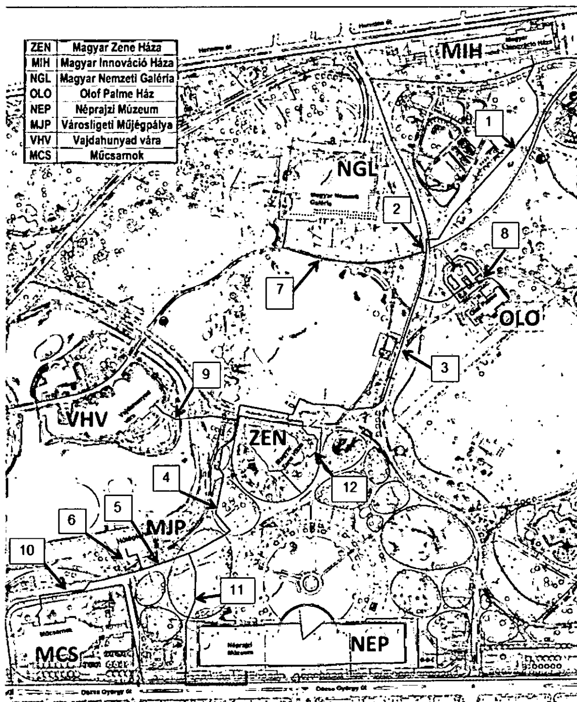
3. ábra Hűtési gerinc vezeték szakaszok
