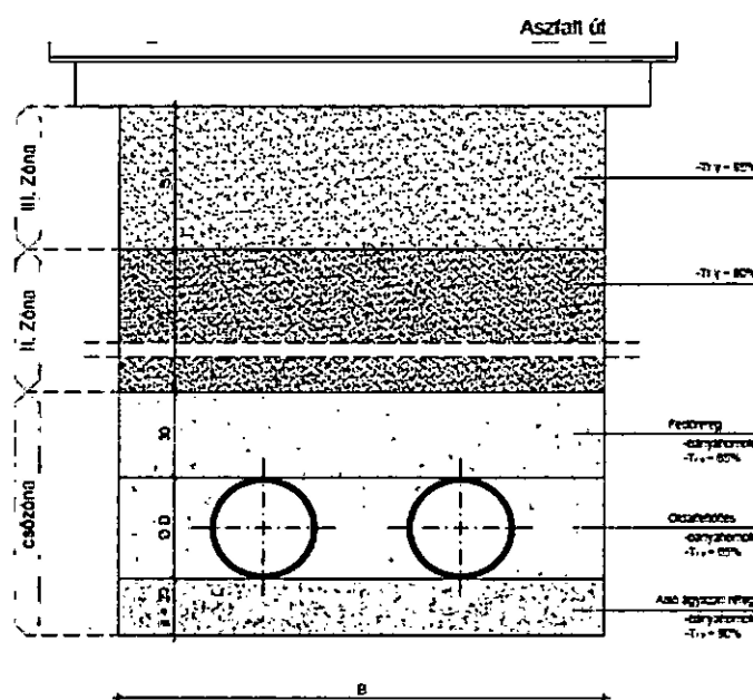
4. ábra SDR17 típusú hűtővezeték ágyazása
