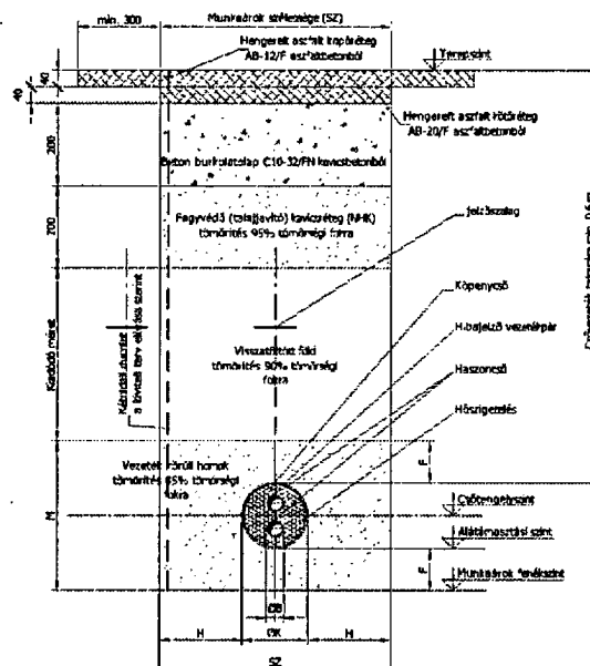
Távfűtési vezeték közút alatti szelvénye Építési követelmény
