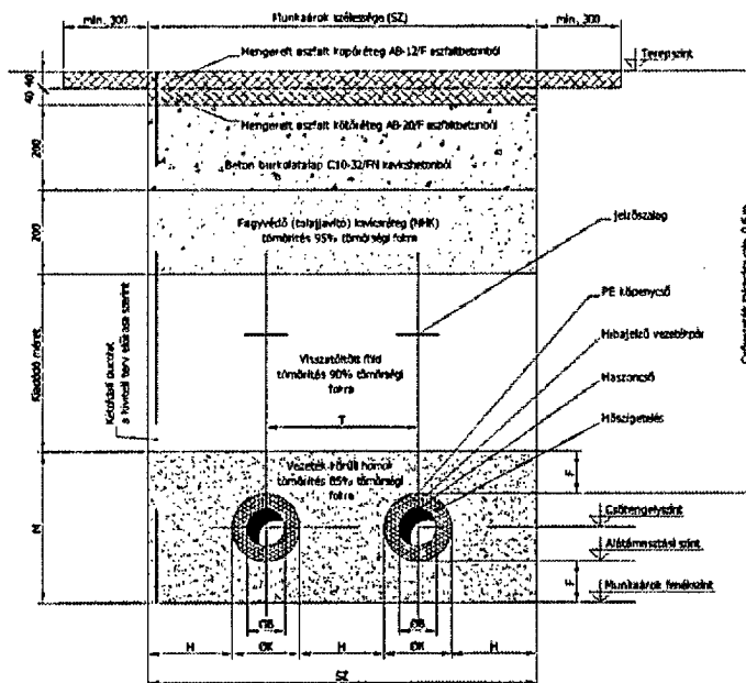
Távfűtési vezeték közút alatti szelvénye Építési követelmény
