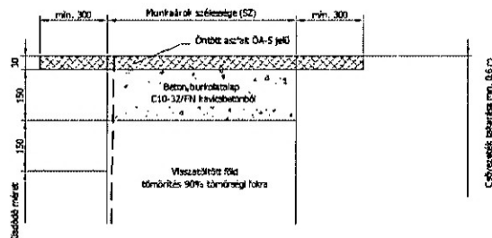
Távfűtési vezeték közút alatti szelvénye Építési követelmény
