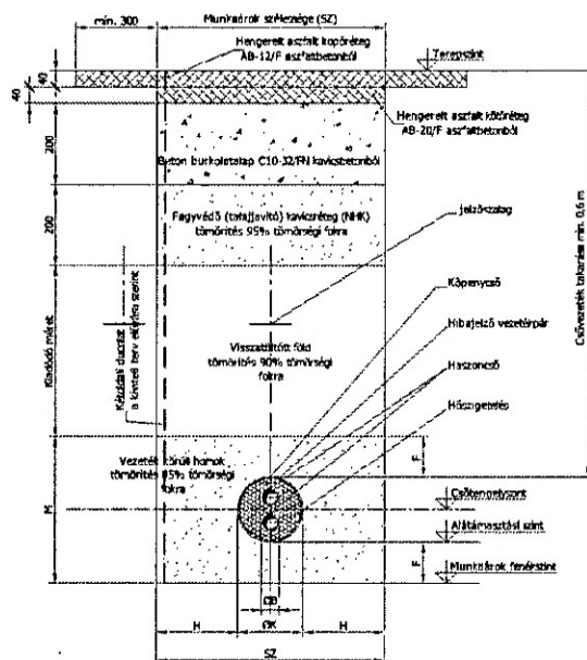
Távfűtési vezeték közút alatti szelvénye Építési követelmény
