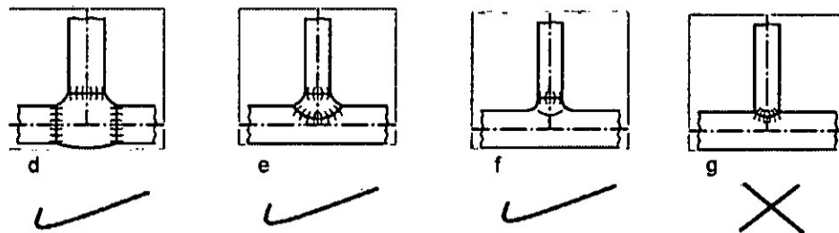
3. ábra: a hegesztett elágazó idomok megengedett kialakítása az MSZ EN 448:2016 szabvány alapján
