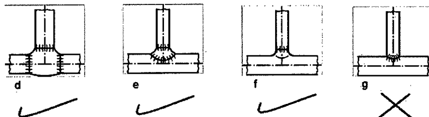
2.ábra: a hegesztett elágazó idomok megengedett kialakítása az MSZ EN 448:2016 szabvány alapján
