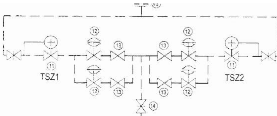
1. ábra: Jelenlegi túláramszelep (TSZ1, TSZ2) kapcsolása
