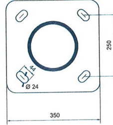
6-9 MÉTERES OSZLOPOKHOZ
